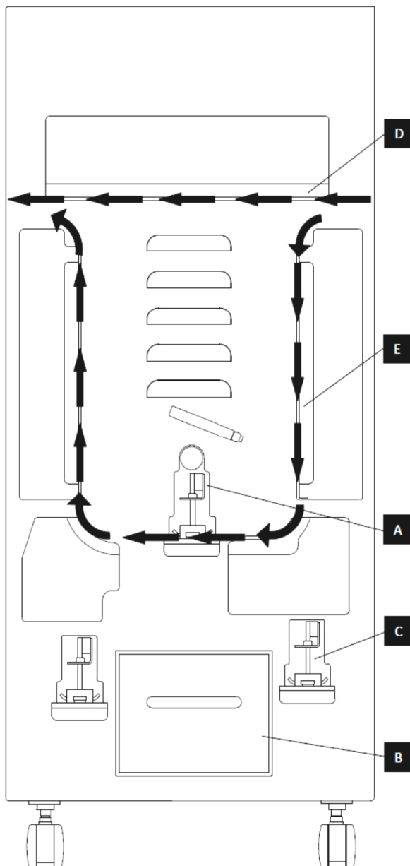
Papierführung und interaktive Bedienerbereiche des PUNCHalfa Plus
