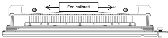
Figura 8.4 Sostituzione della barra di pressione
