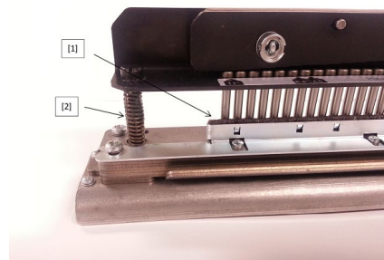
Abbildung 8.8 Schmierung
