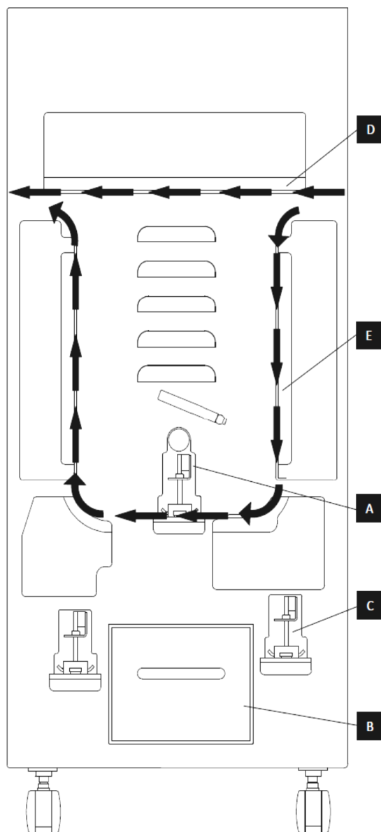
Flujo del papel y secciones Interactivas de Usuario de la PUNCHalfa Plus
