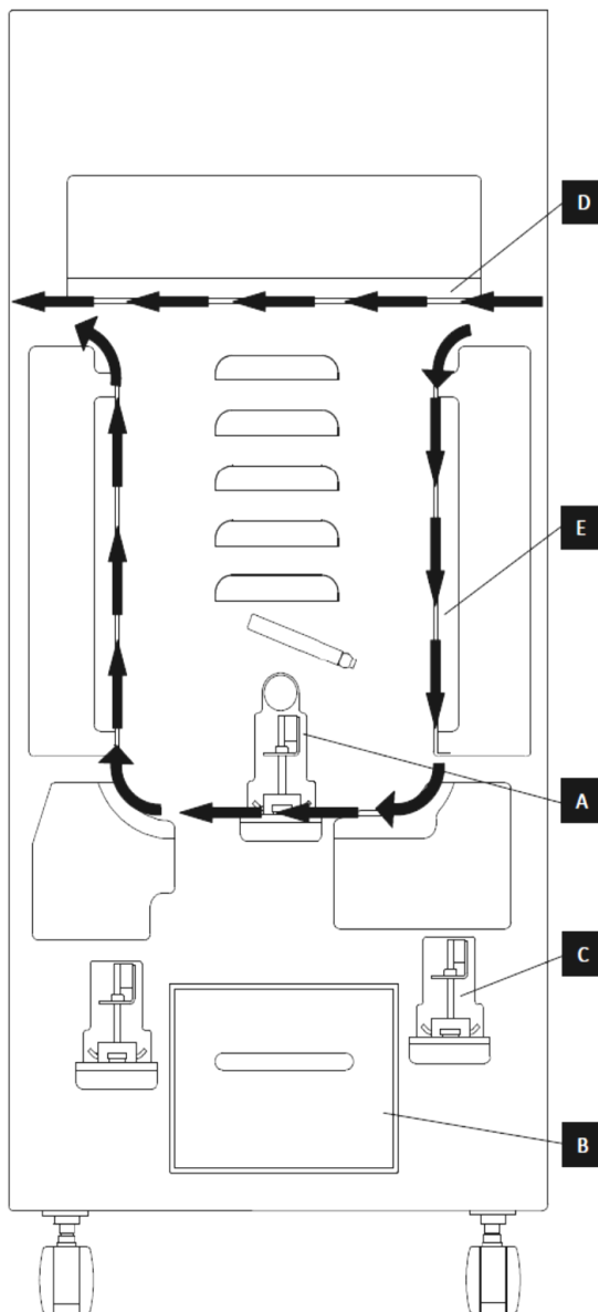
Flujo del papel y secciones Interactivas de Usuario de la StreamPunch Plus
